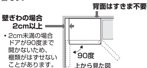
図は必要最小設置寸法です。(消費電力量測定時の寸法とは異なります)
