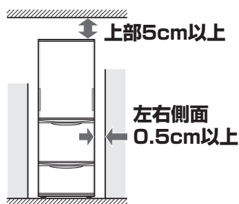
図は必要最小設置寸法です。(消費電力量測定時の寸法とは異なります)
