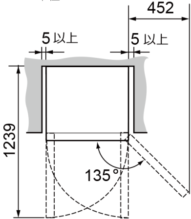
据え付けスペース ・単位：mm
