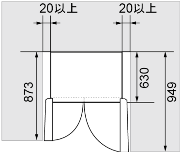
据え付けスペース ・単位：mm
