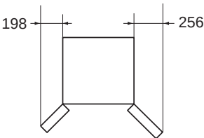
135° 開時の寸法
