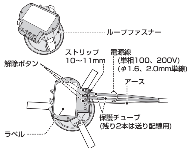
電源線接続例 (保護チューブを使用する場合)
