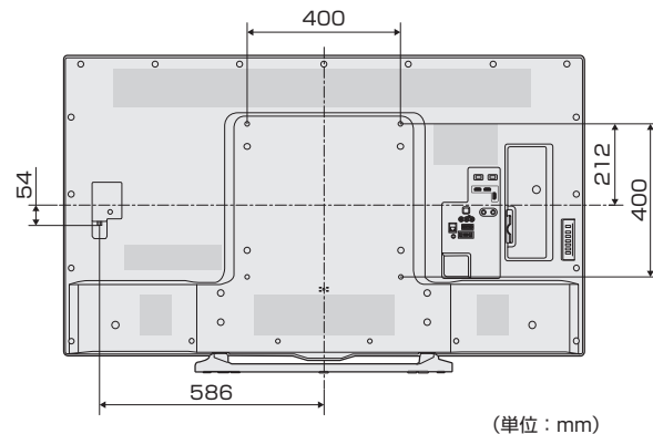
壁掛け金具取り付け部の寸法
