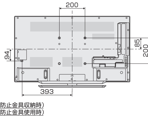
壁掛け金具取り付け部の寸法
