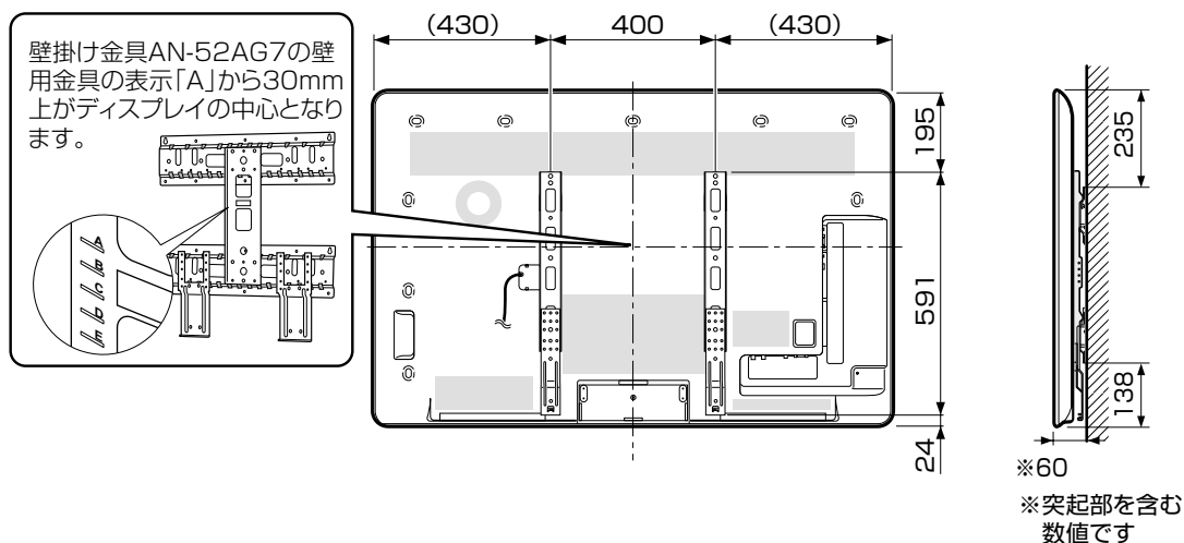
壁掛け金具AN-52AG7使用時
