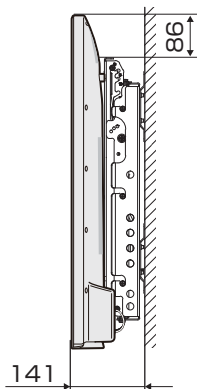
壁掛け金具AN-52AG6使用時
