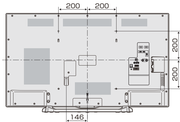
壁掛け金具取り付け部の寸法
