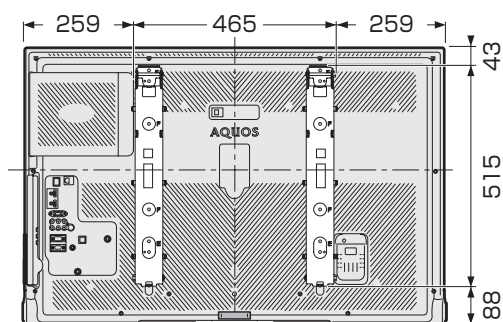
壁掛け金具AN-52AG6使用時
