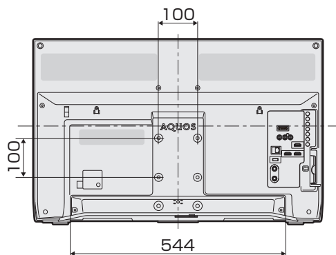
壁掛け金具取り付け部の寸法
