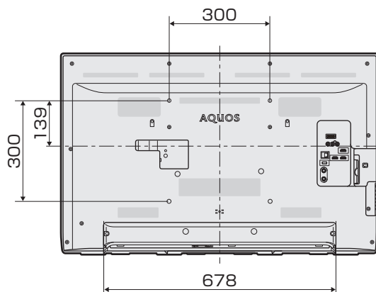
壁掛け金具取り付け部の寸法
