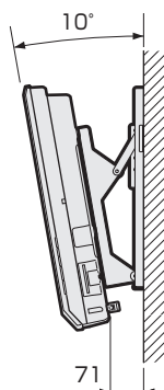
壁掛け金具AN-37AG3使用時
