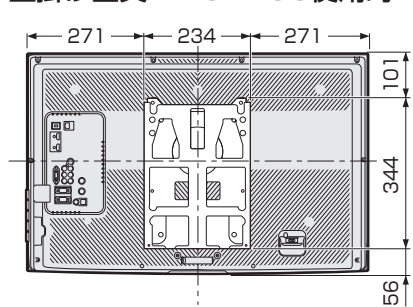
壁掛け金具AN-37AG3使用時
