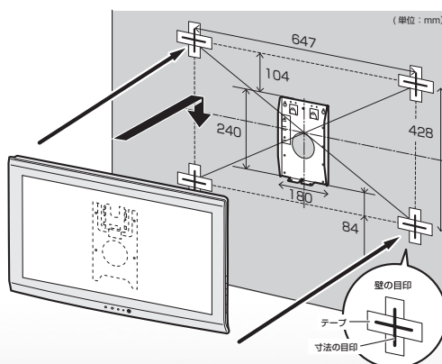
壁掛け金具 AN-130AG1 使用時
