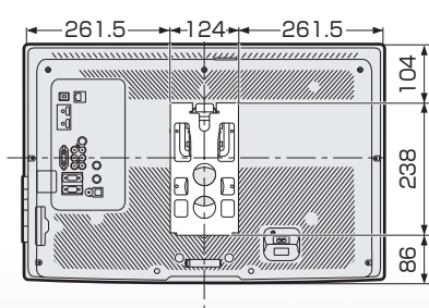
壁掛け金具AN-130AG1使用時
