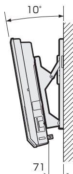
壁掛け金具AN-37AG3使用時
