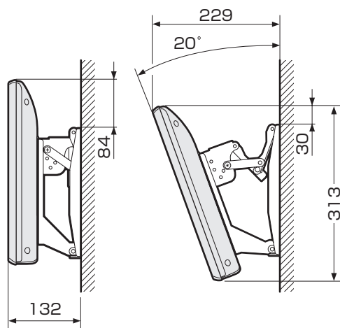
壁掛け金具AN-130AG1使用時
