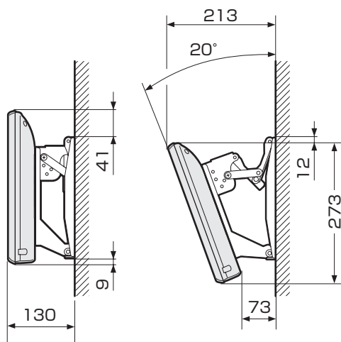
壁掛け金具AN-130AG1使用時
