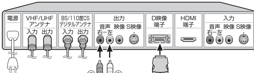
D映像ケーブル (市販品) 音声ケーブル (市販品)
