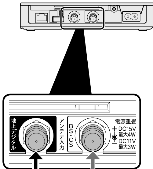
▼チューナー一部背面
