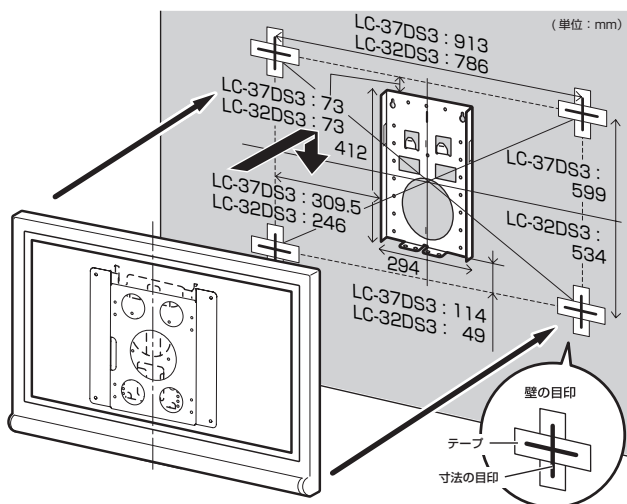
壁掛け金具 AN-37AG2 使用時
