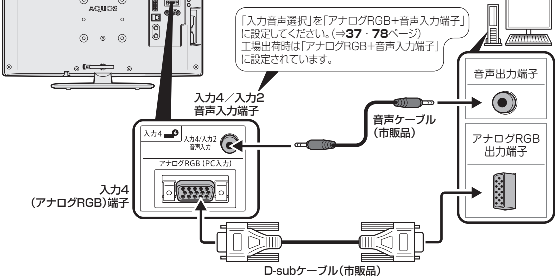
本体背面
