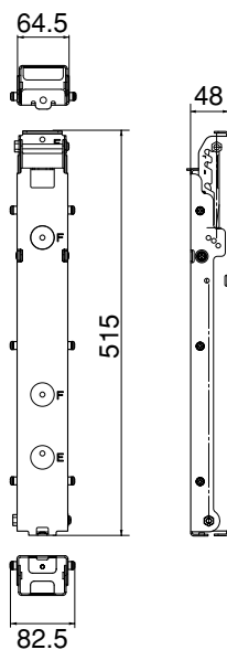
壁掛け金具ユニット (左/右)
