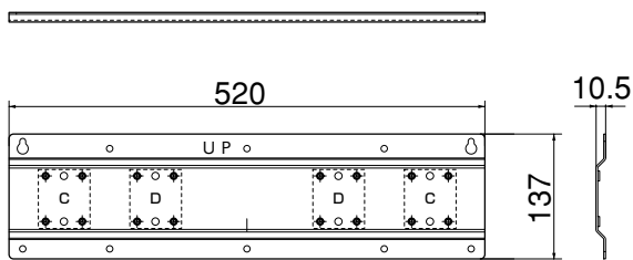
壁用金具 B
