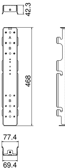
壁用金具 B
