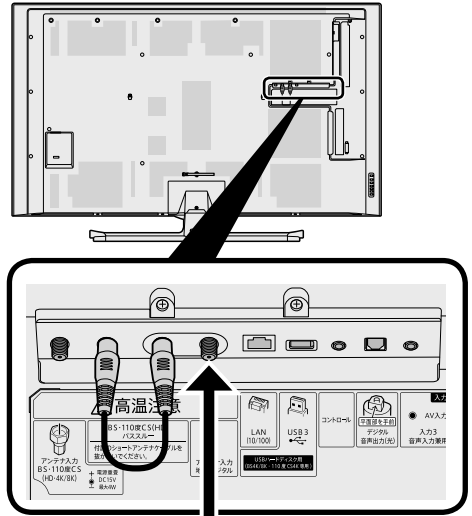
▼本体背面
