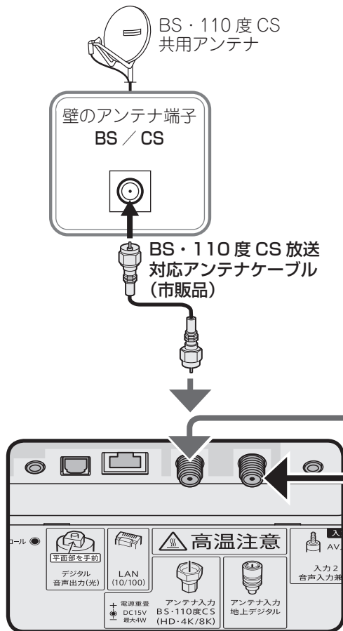
◀本体背面端子部
