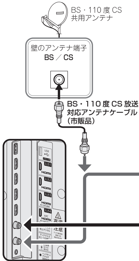
◀本体背面端子部
