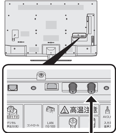
▼本体背面
