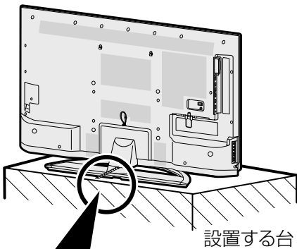
市販のワッシャーネジ
