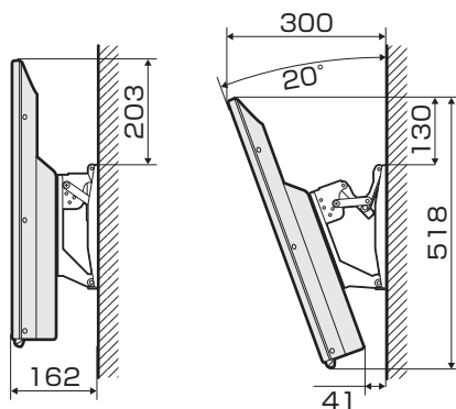
壁掛け金具AN-130AG1使用
