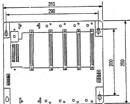
増設ベースユニット (ZW-104ZB)
