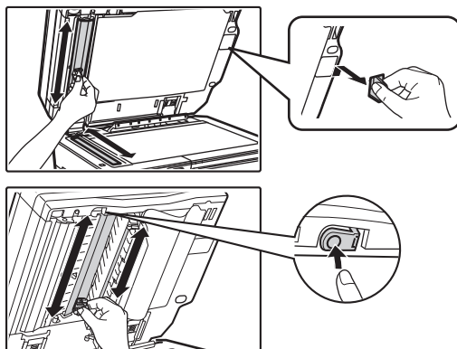
両面原稿同時自動送り装置（DSPF）の場合
