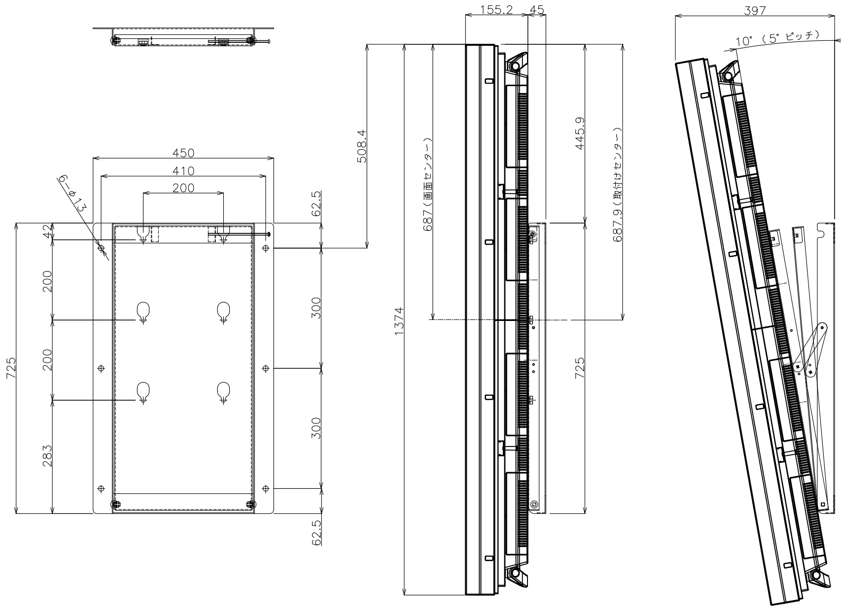
壁掛け金具 (PN-A601: 保護ガラス付 取付時) PN-ZK602 外観図
