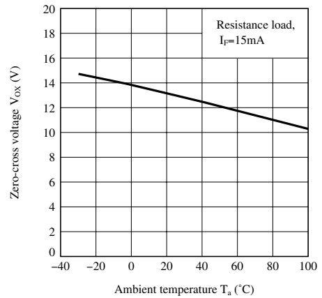
Fig.10-a ゼロクロス電圧 周囲温度特性 (ランクB)
