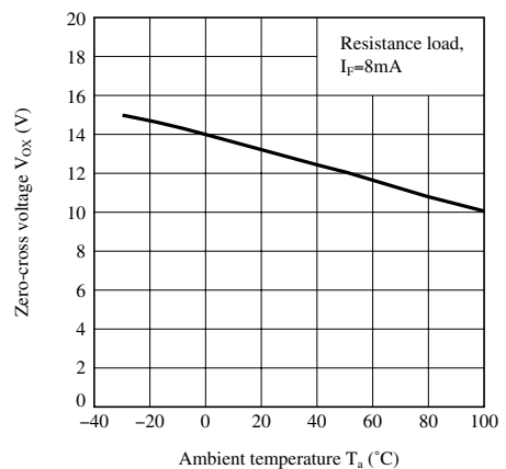
Fig.10 ゼロクロス電圧 周囲温度特性
