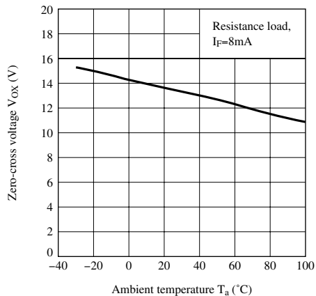
Fig.10-b ゼロクロス電圧 周囲温度特性 (ランクC, ランクD)
