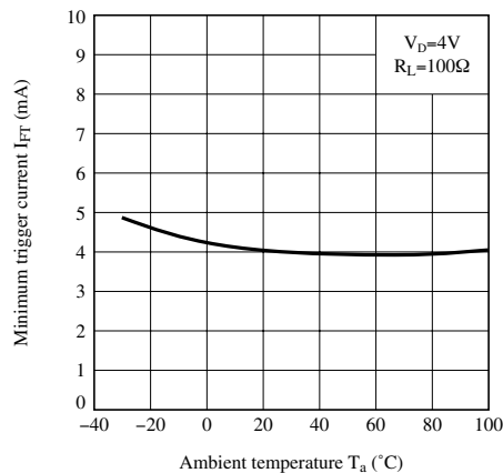
Fig.4-a 最小トリガー電流 周囲温度特性(ランクB)
