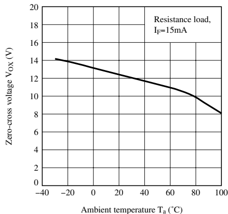
Fig.10-a ゼロクロス電圧 周囲温度特性 (ランクB)
