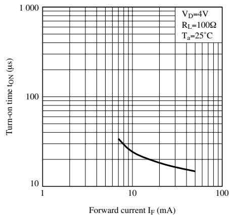
Fig.9-a ターンオン時間 順電流特性 (ランクB)
