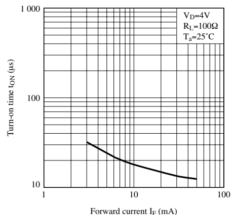
Fig.9-a ターンオン時間 順電流特性 (ランクC, ランクD)
