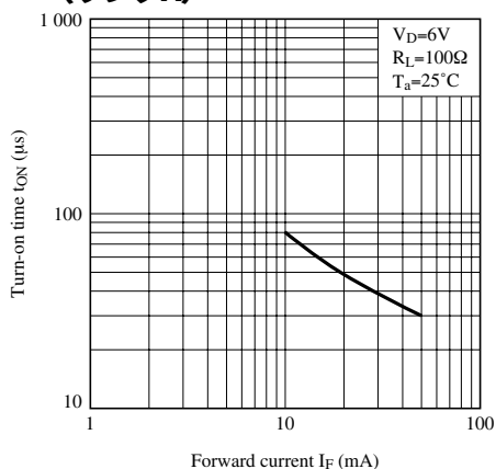
Fig.9-a ターンオン時間—順電流特性 (ランクA)
