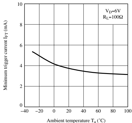
Fig.4-b 最小トリガー電流—周囲温度特性 (ランクB、ランクC)
