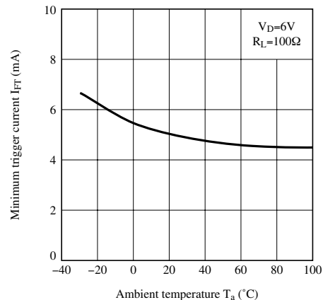
Fig.4-a 最小トリガー電流—周囲温度特性 (ランクA)
