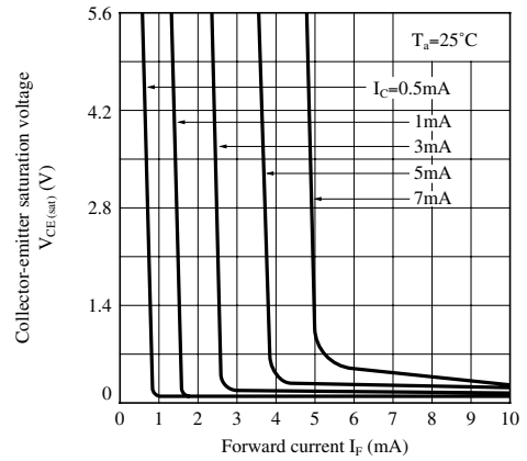
Fig.14 コレクタ・エミッタ間飽和電圧 順電流特性
