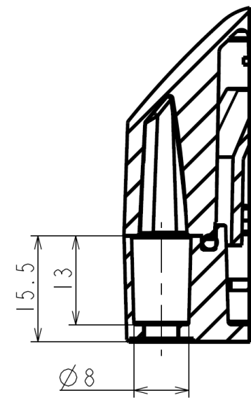
SEC. A-A S=1:1 (3箇所)
