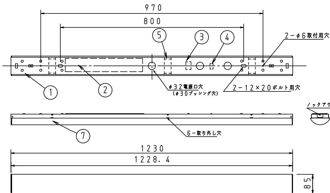
側面詳細図
