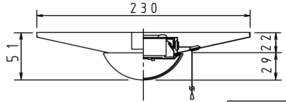
側面詳細図
