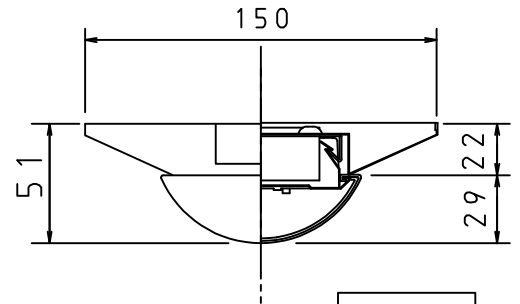
側面詳細図
