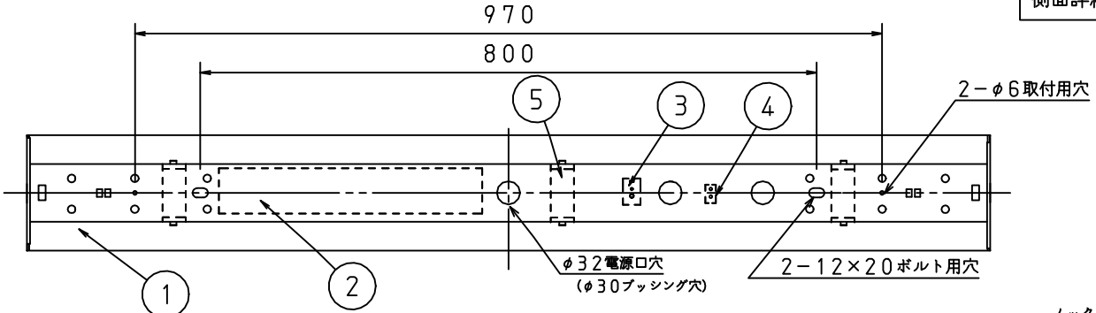
側面詳細図
