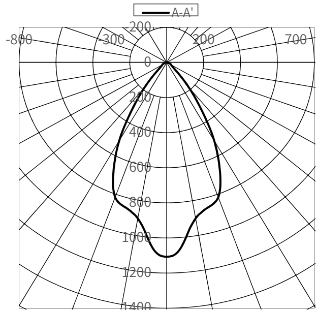
配光曲線(cd/1,000Lm)
