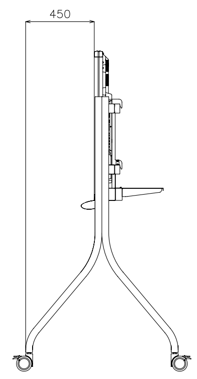
フロアスタンド (PN-L702B取付時) PN-ZS70F 外観図
