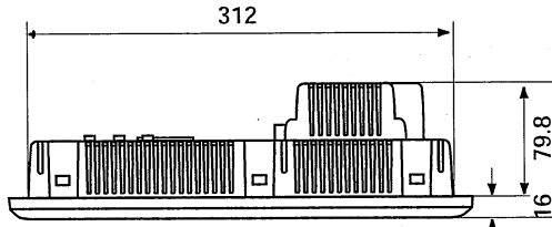
○上面図
