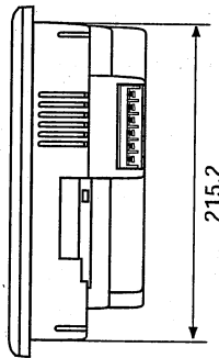
○側面図
