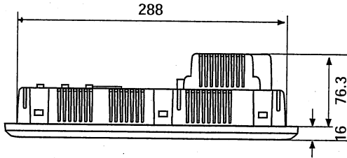
○上面図
