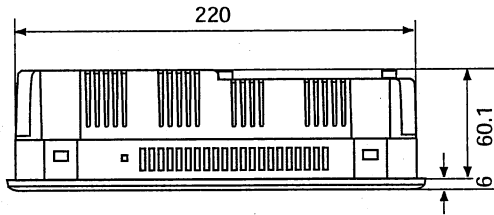
○上面図
